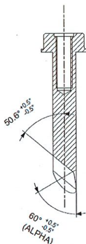
SEZ. A-A
